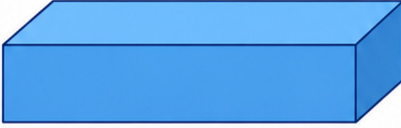
Dikdörtgen prizma
