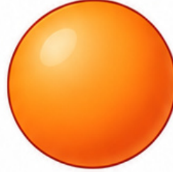
Küre
