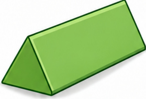
Üçgen prizma
