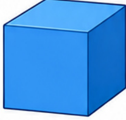
Küp
