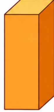
Kare prizma
